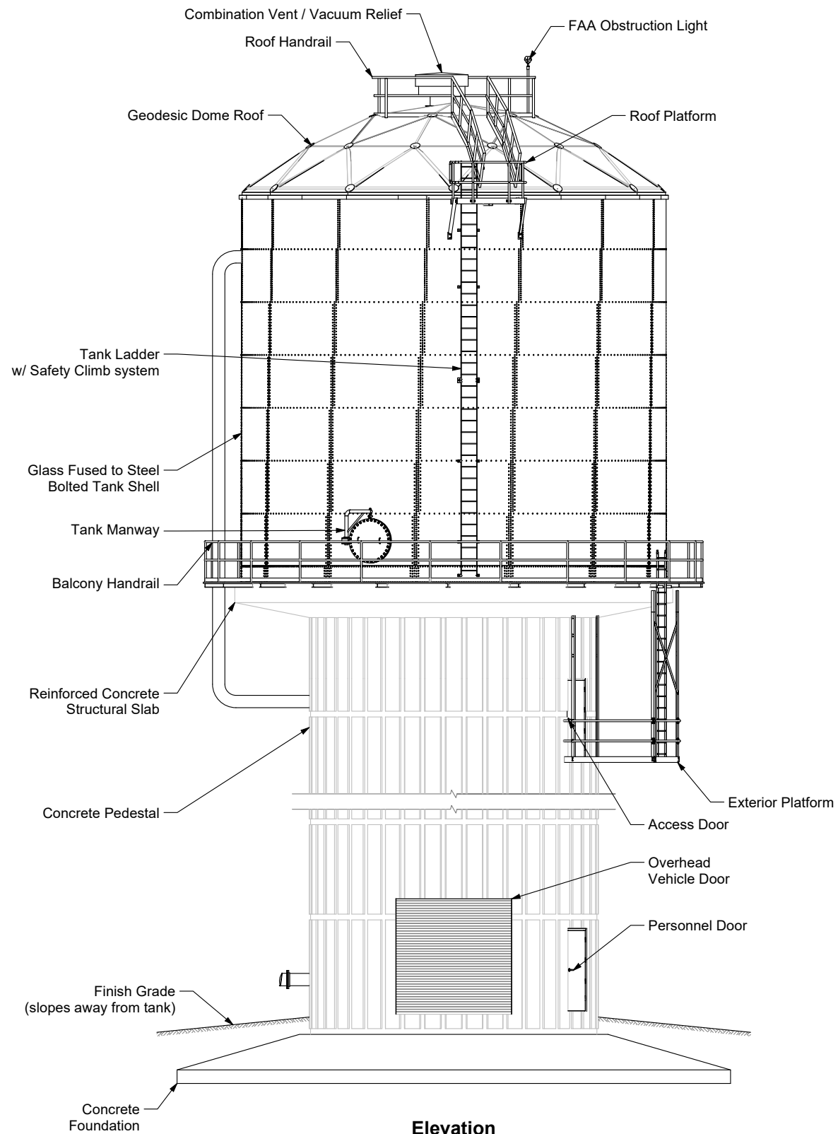
Elevation
